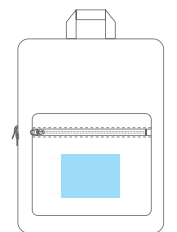
シルク: W120×H90mm
